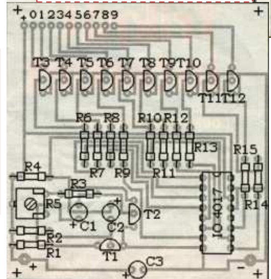
Rozmístění součástek na jedné desce
